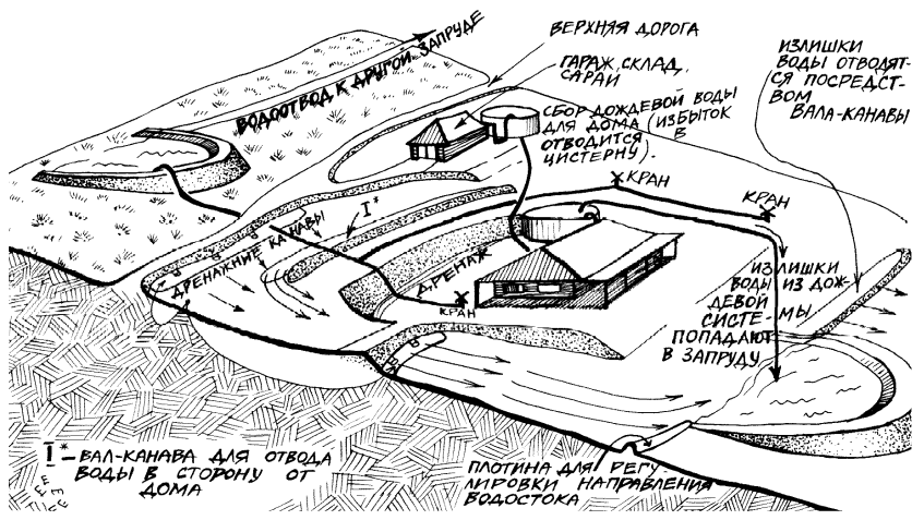
Рис. 2. Идеальный пример взаиморасположения систем водоснабжения, строений и дорог. Валы-канавы служат для отвода воды по горизонталям склона, что способствует уменьшению степени эрозии во время выпадения обильных осадков.
